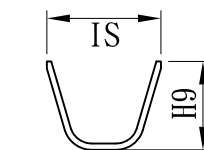
A-A Section
