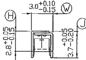
SEC.B-B
