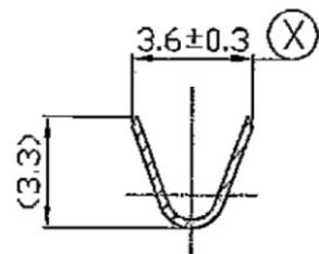
SEC.A-A
