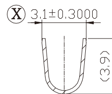
SEC.A-A
