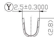
SEC.B-B
