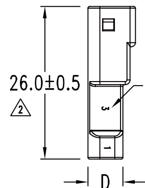
SEC. A-A
