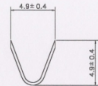
A-A Section
