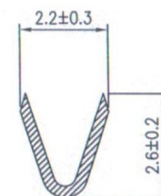
A-A SECTION
