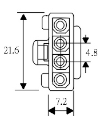
PSL-S-1X04
