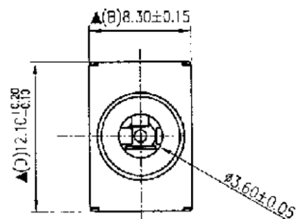
視圖 A(2:1)
