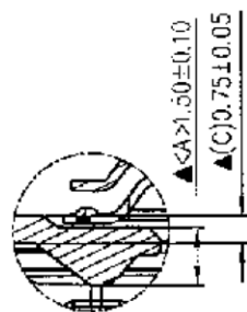
視圖 A(2:1)
