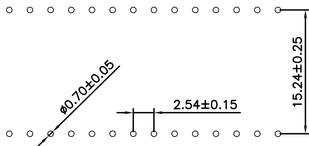
P.C.B LAYOUT
