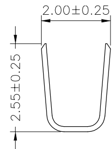
SEC:A-A
