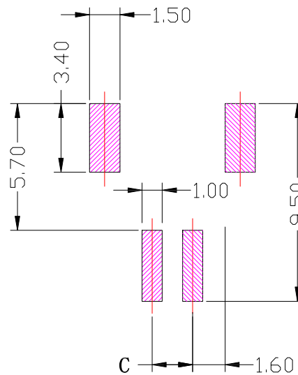
P.C.B Hole Layout
