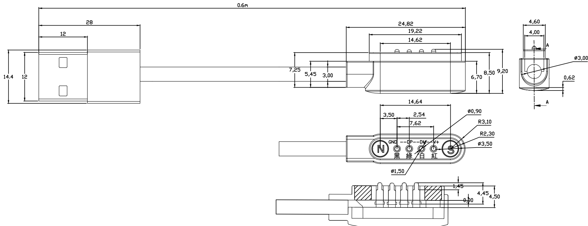
剖面 A-A
