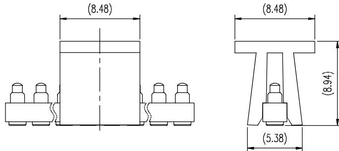
Cap Option(4 Pins ~ 16 Pins) Scale: 2:1
