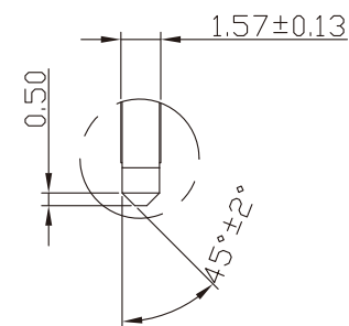
DETAIL:A SCALE :2:1
