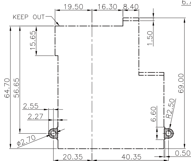
PCB LAYOUT( TOL ±0.05)
