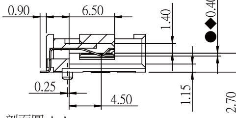
剖面圖 A-A
