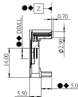
A-A (1.3 : 1)
