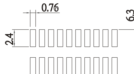
P.C.Board Layout
