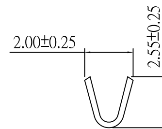
A-A SECTION
