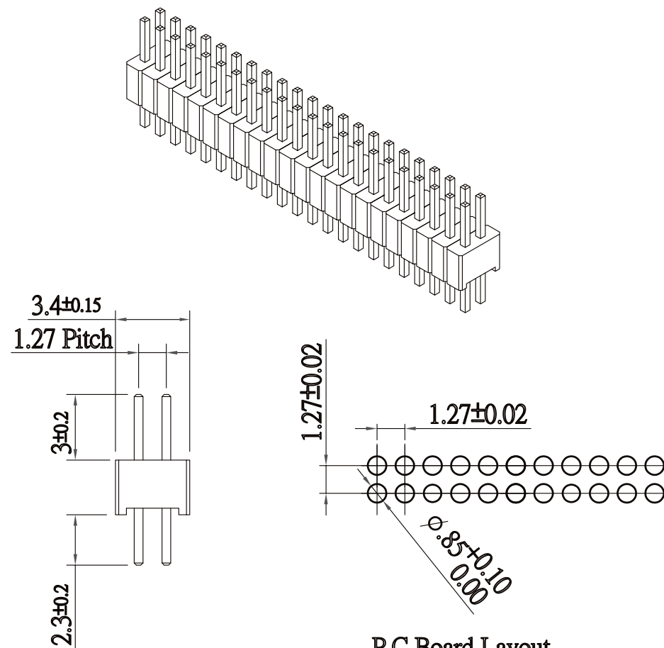
P.C.Board Layout
