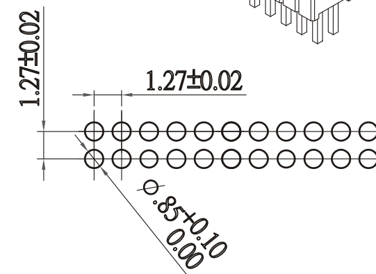
P.C.Board Layout
