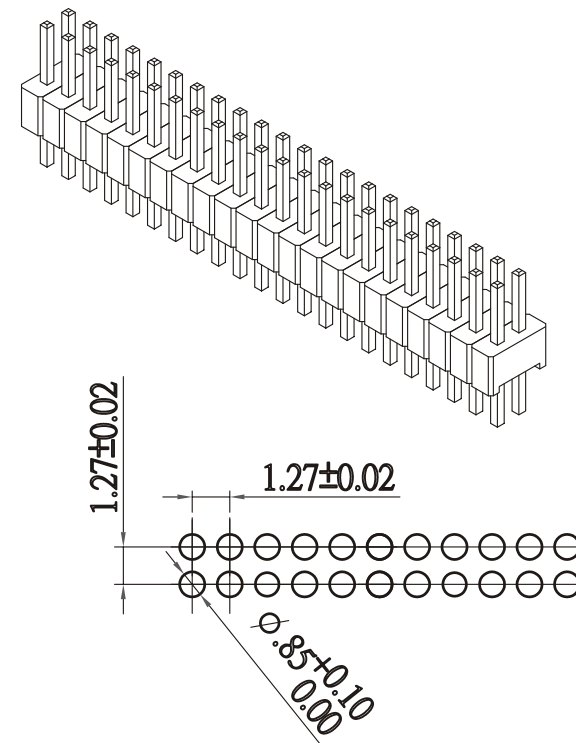
P.C.Board Layout
