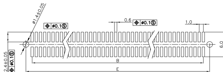
P.C.Board Layout
