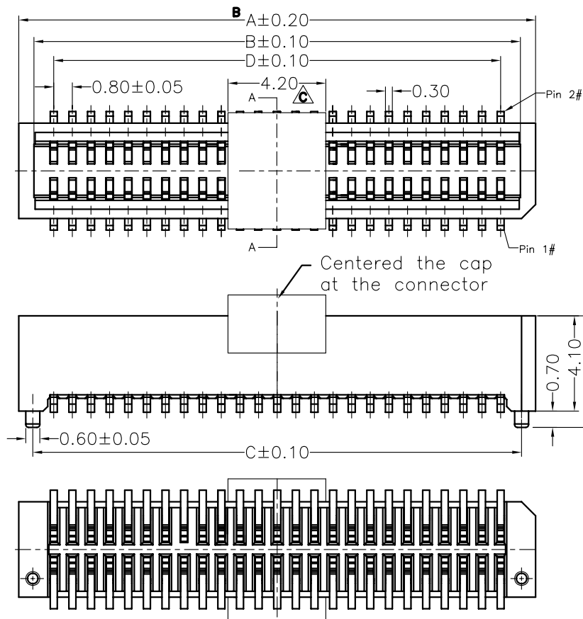
Contacts Dimensions :
