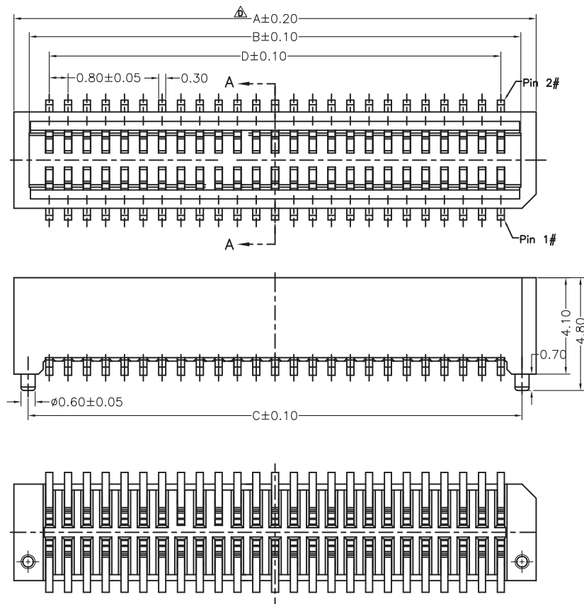
Contacts Dimensions :
