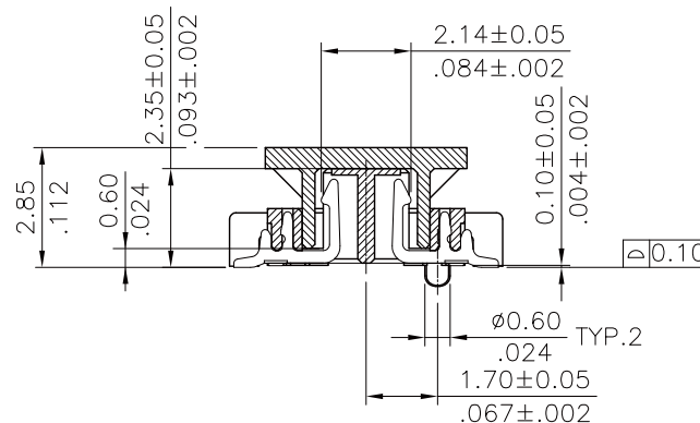
A-A SEC.
