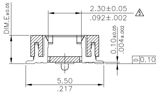
A-A SEC.
