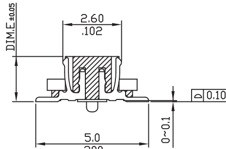
A-A SEC
