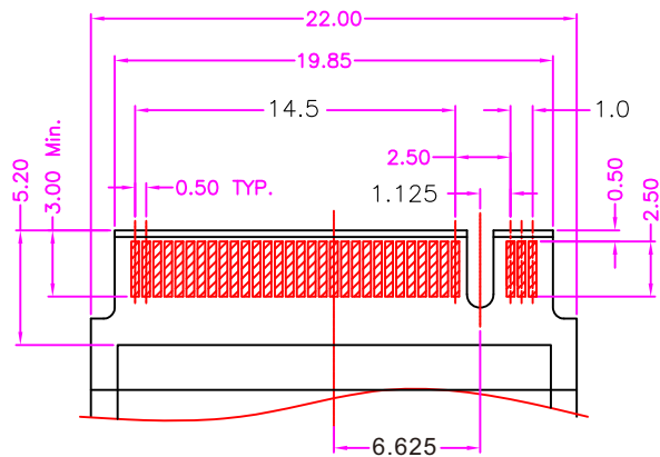
BOTTOM SIDE
