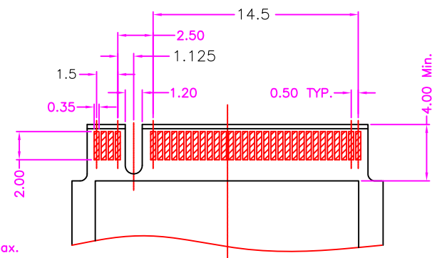
TOP SIDE
