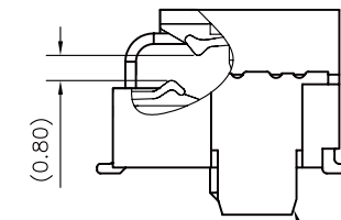
SECTION A-A(SCALE 4:1)
