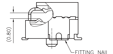
SECTION A-A Scale 4:1
