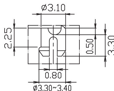
DETAIL Y
