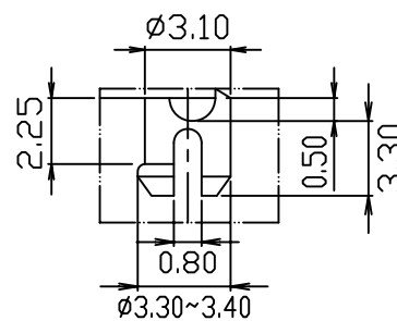
DETAIL Y
