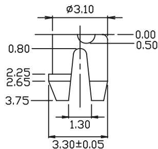
DETAIL Y
