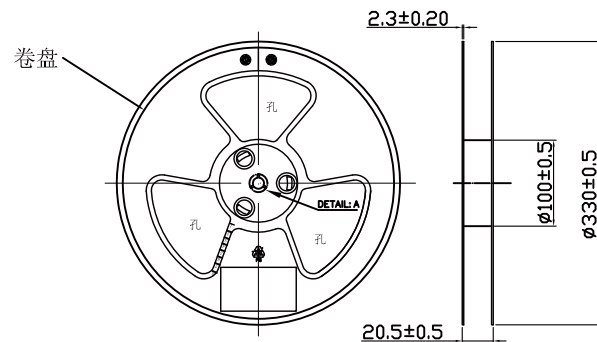
卷帶盤 (圖一)
