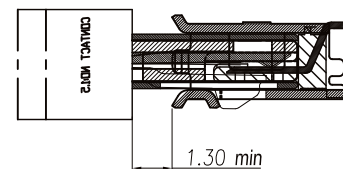
公母插内部結構圖
