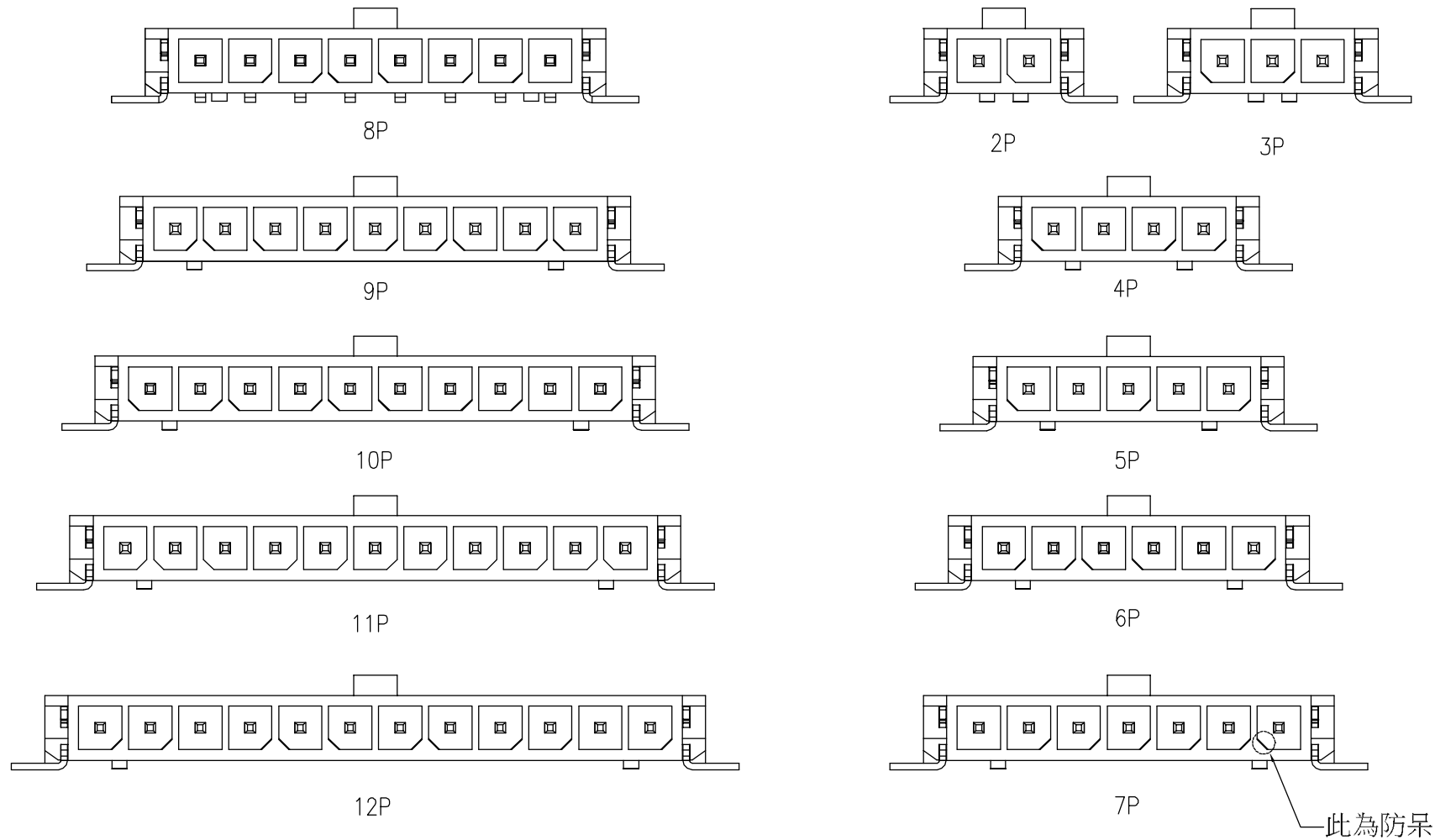
2-12 Pin防呆位置分部示意图
