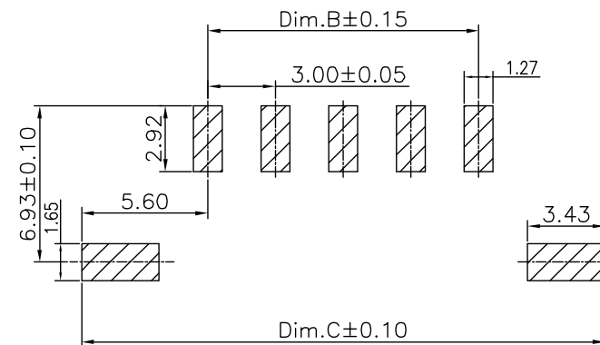
P.C.B Layout
