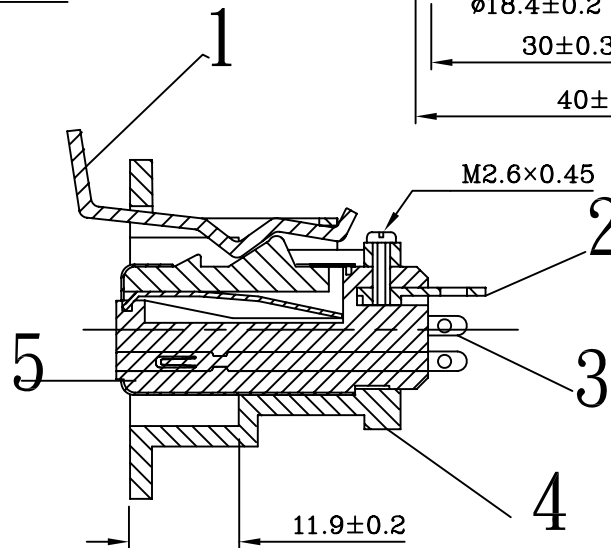
A-A SECTION
