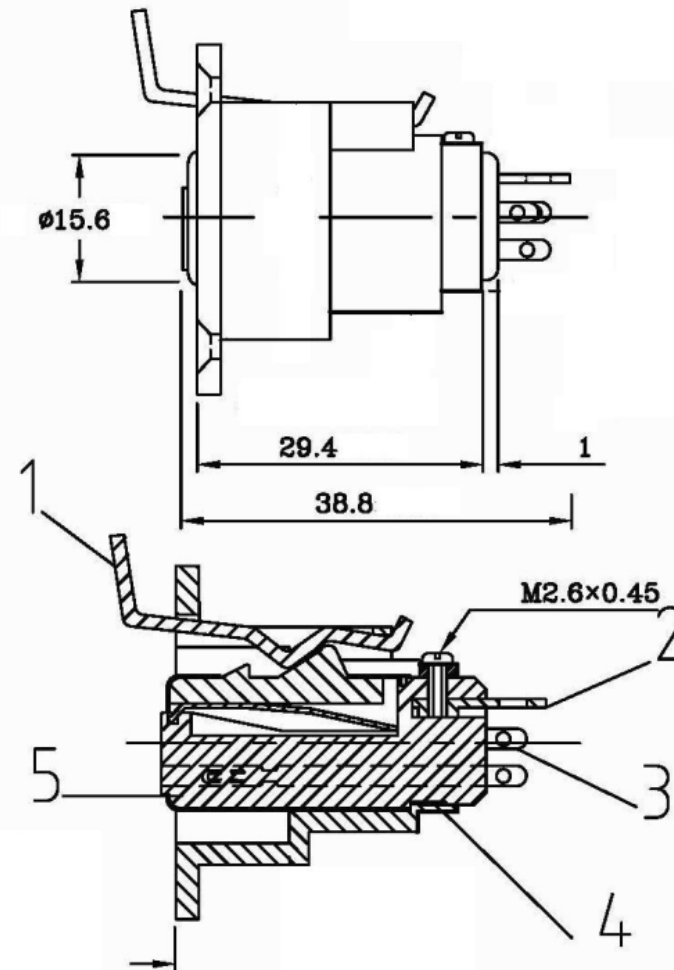
A-A SECTION
