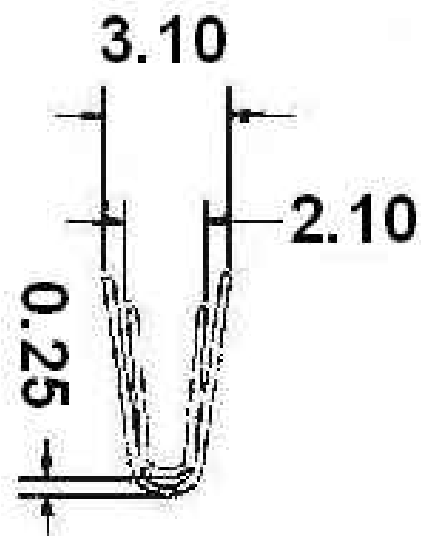
A-A Section
