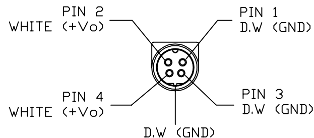
4P POWER DIN FRONT VIEW
