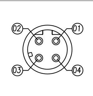
Pin 前視圖
