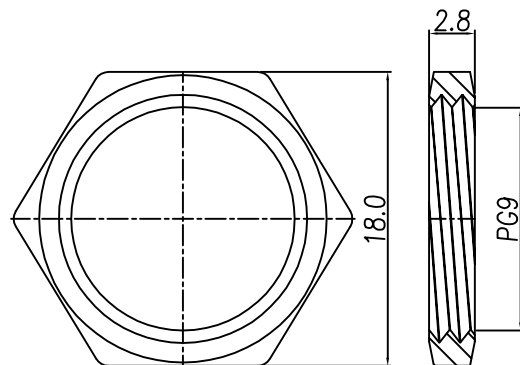
NUT
