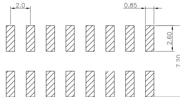
P.C.B Layout
