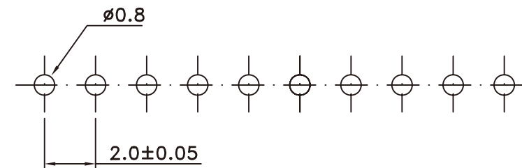
P.C.B. LAYOUT
