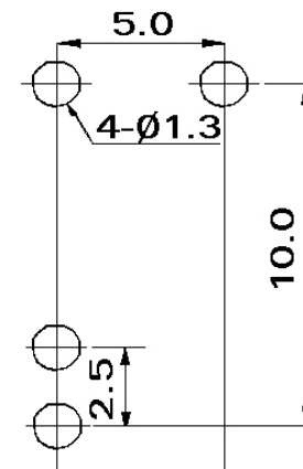
P.C.B. LAYOUT
