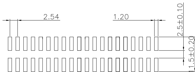
P.C.B Layout
