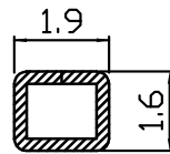
SECTION D-D
