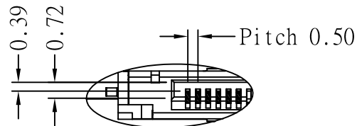
DETAIL-A SCALE 2.5:1
