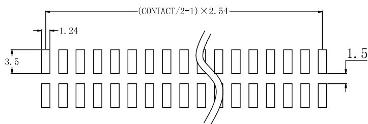
P.C.B . LAYOUT
