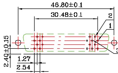
2N P.C.Board Hole Pattern
